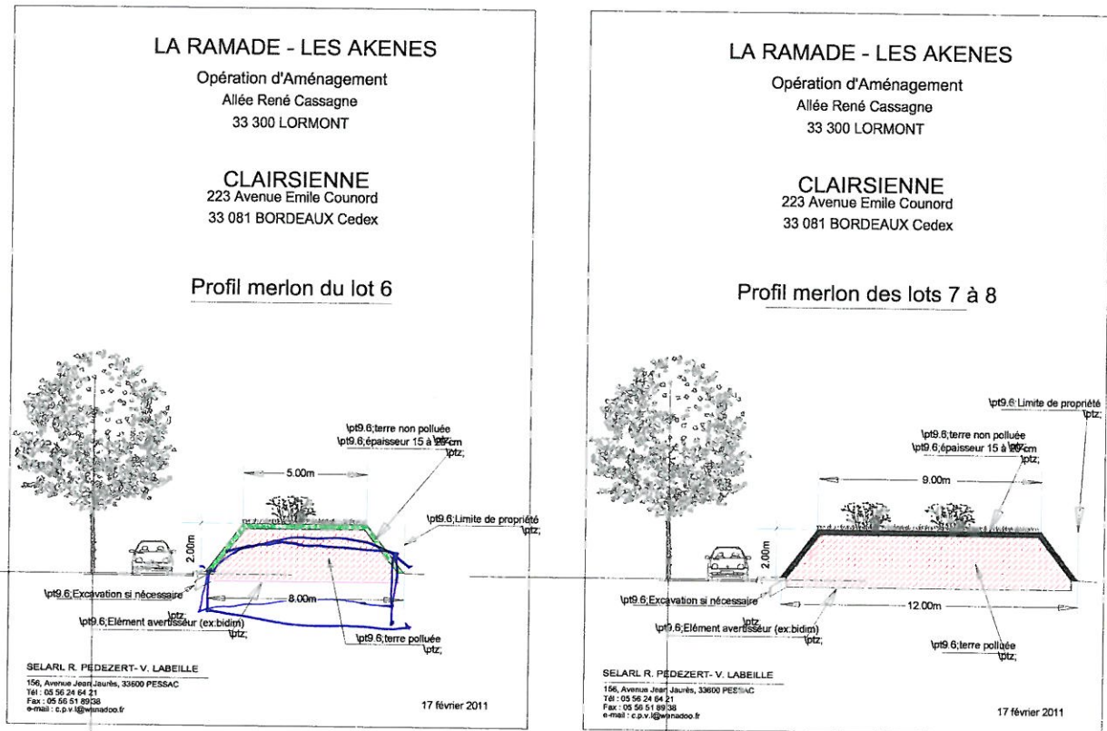
Figure n°5 : Coupe schématique des merlons. 05.043.CO.005.1,fig5
